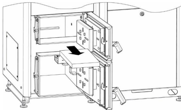
KROK 2: Ostrożnie unieść płytę górną i wysunąć z kotła.
