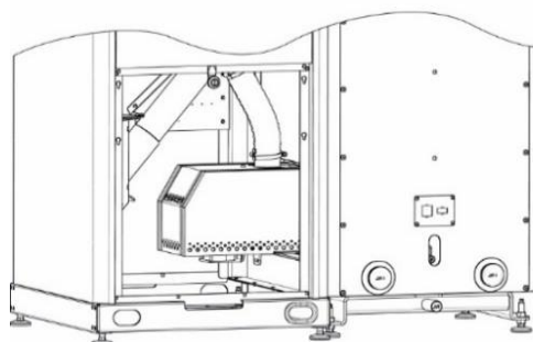
Rysunek 6. Prawidłowe ułożenie rury i ustawienie zasobnika.
