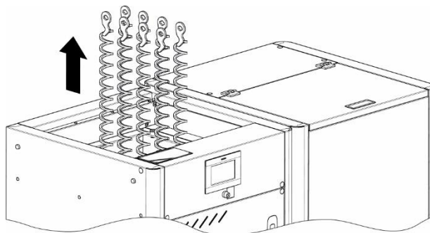
KROK 5. Ostrożnie wysunąć zawleki z rury płomieniowej, oczyścić; ponowny montaż wykonać w odwrotnej kolejności
