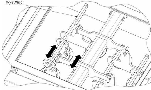
KROK 4. Przesuwając ramię oraz belki mechanizmu systemu automatycznego zdemontować zawleki.
