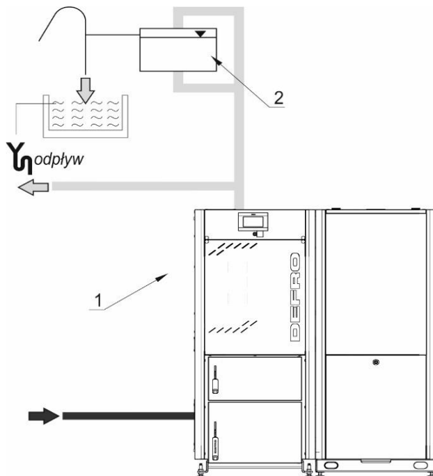
Rysunek 7. Przykładowy schemat zabezpieczeń kotła GAMMA II w układzie otwartym:
