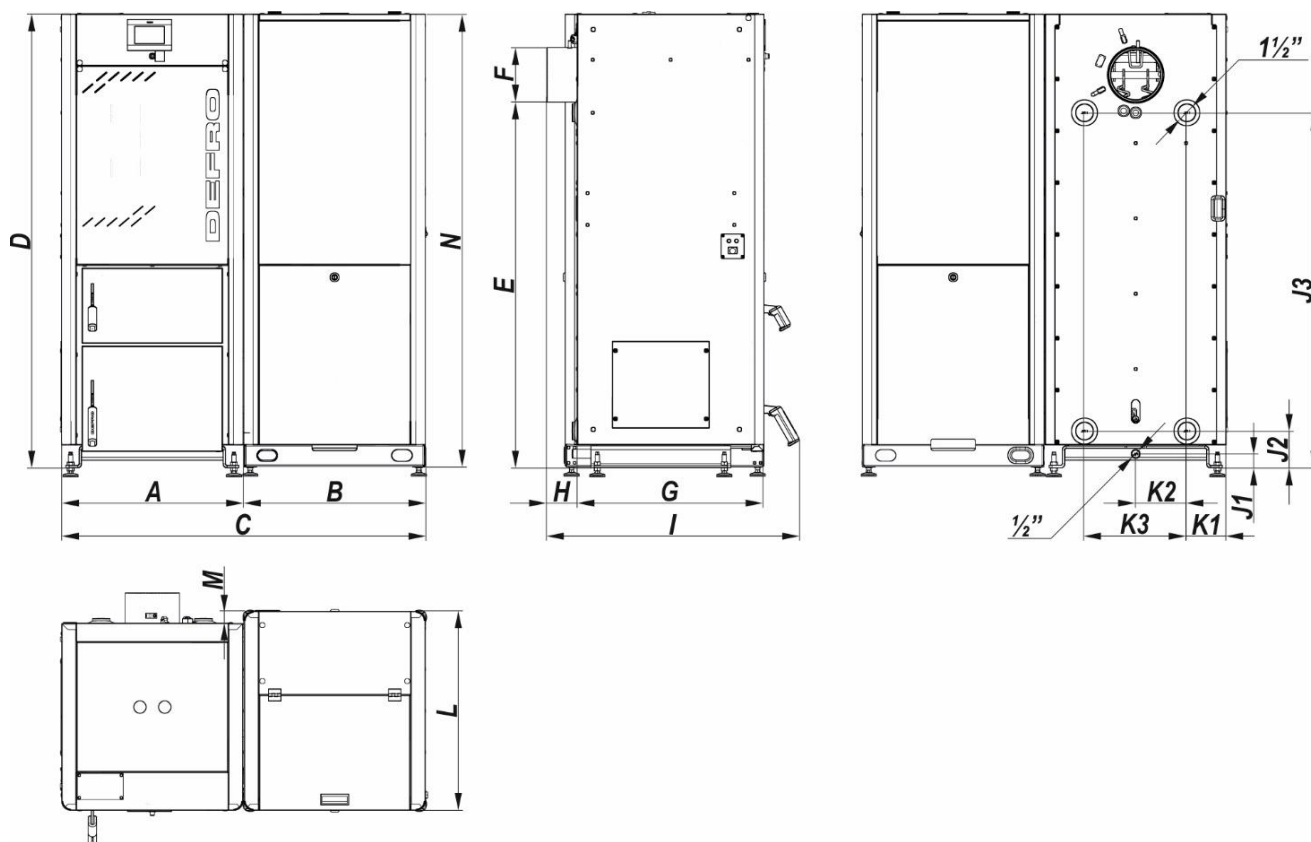
Rysunek 2. Podstawowe wymiary kotłów GAMMA II
