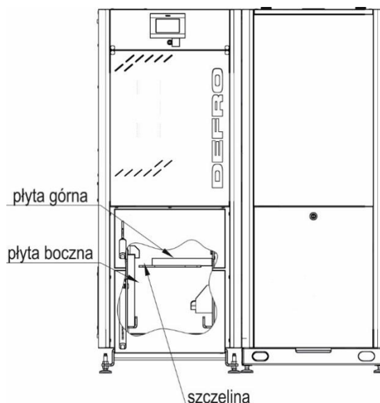
Rysunek 1. Rozmieszczenie katalizatorów ceramicznych w kotle, wersja ze zbiornikiem z prawej strony
