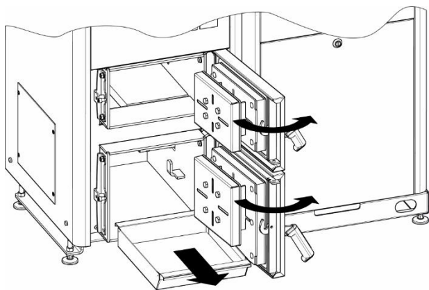
KROK 1: Otworzyć drzwi kotła, usunąć z kotła szufladę popielnika
