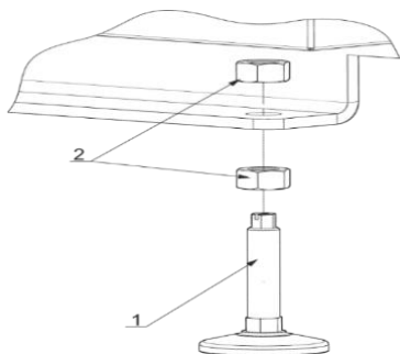
Rysunek 4. Regulowane stopki kotła.
