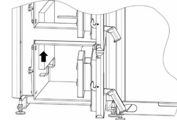
KROK 4: Ostrożnie zdjąć płytę boczną z uchwytów.
