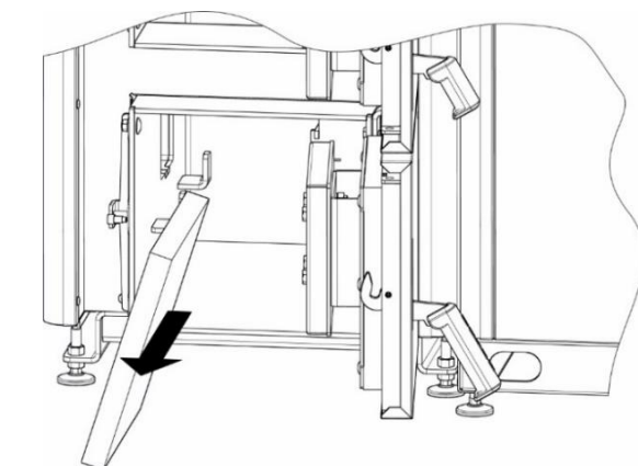
KROK 5: Wysunąć płytę ceramiczną z kotła. Oczyszczyć ściany komory paleniskowej kotła. Ponownie umieścić płyty ceramiczne w kotle postępując w odwrotnej kolejności.
