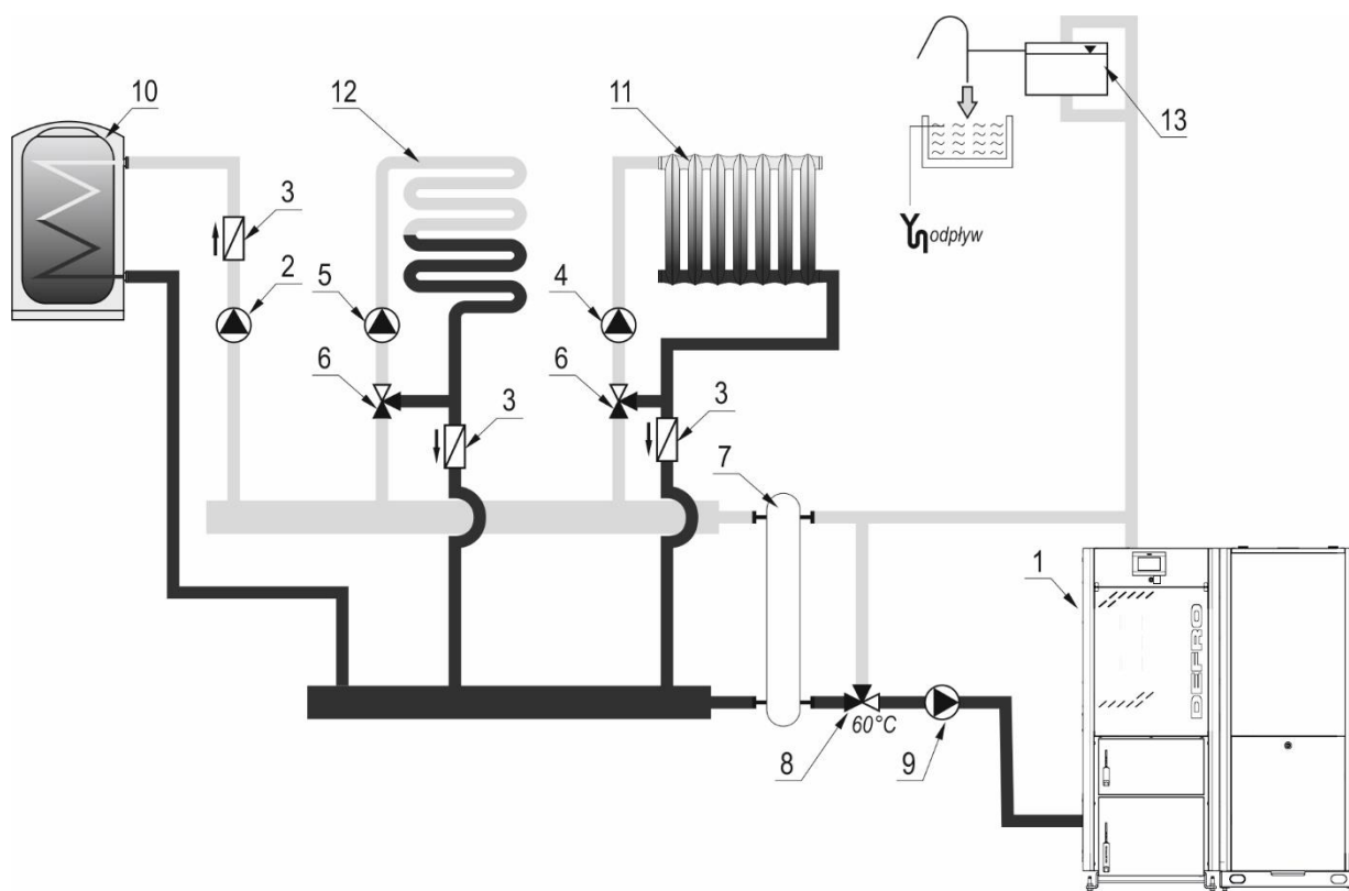
Rysunek 9. Uproszczony schemat instalacji grzewczej systemu otwartego.
