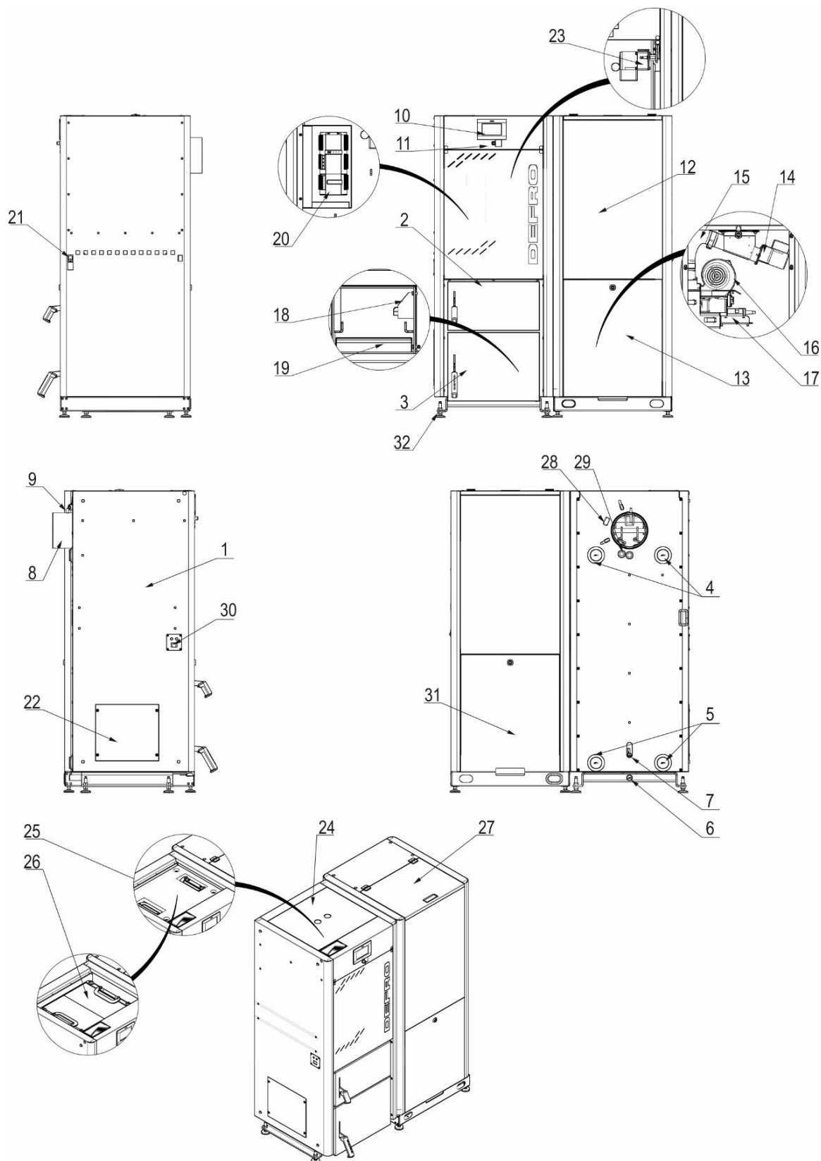
Rysunek 3. Podstawowe elementy kotła GAMMA II
