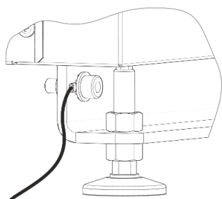
Rysunek 11. Uziemia kotła.
