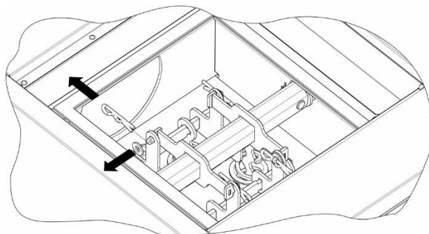
KROK 3. Rozłączyć ramię mechanizmu systemu automatycznego czyszczenia poprzez wypięcie zawlecarki
