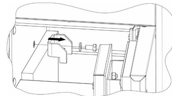
KROK 3: Odkręcić śrubę mocującą płyty ceramiczne
