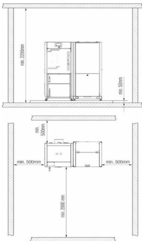
Rysunek 5. Ustawienie kotła w pomieszczeniu kotłowni.
