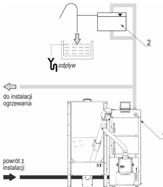
Rysunek 9. Przykładowy schemat zabezpieczeń automatycznego kotła FIREWOOD DUO w układzie otwartym
