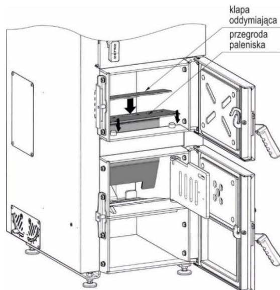
Rysunek 15. Montaż przegrody paleniska
