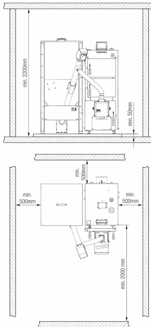
Rysunek 8. Ustawienie kotła w pomieszczeniu kotłowni.
