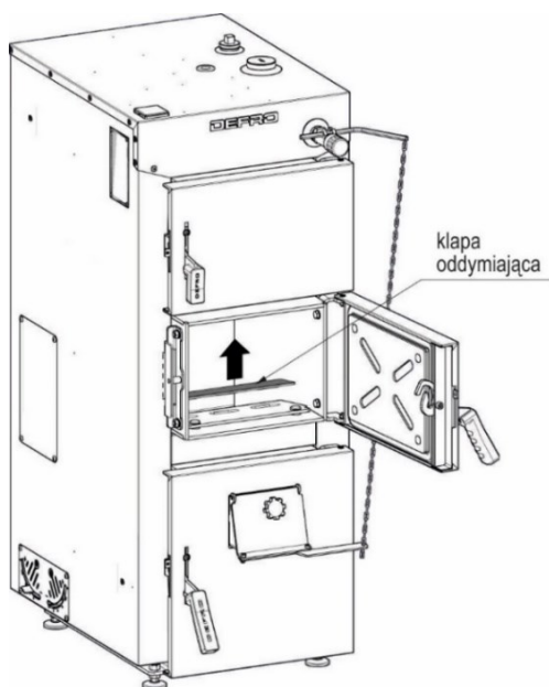
Rysunek 22. Kłapa oddymiająca w przegrodzie paleniskowej.
