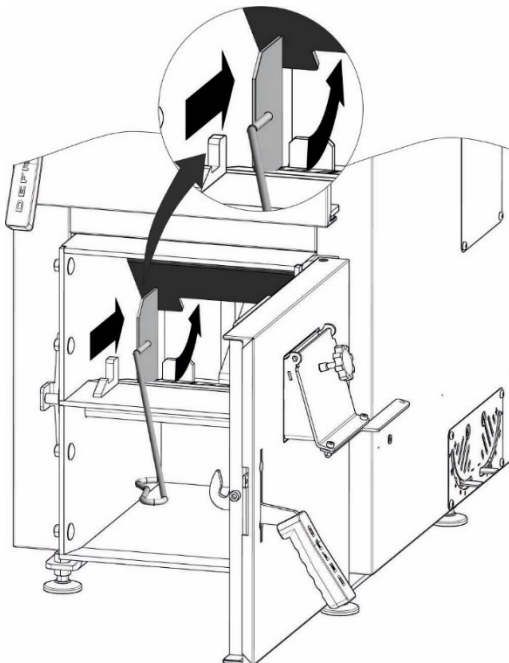
Rysunek 18. Przygotowanie przegrody paleniska do rozpalania.
