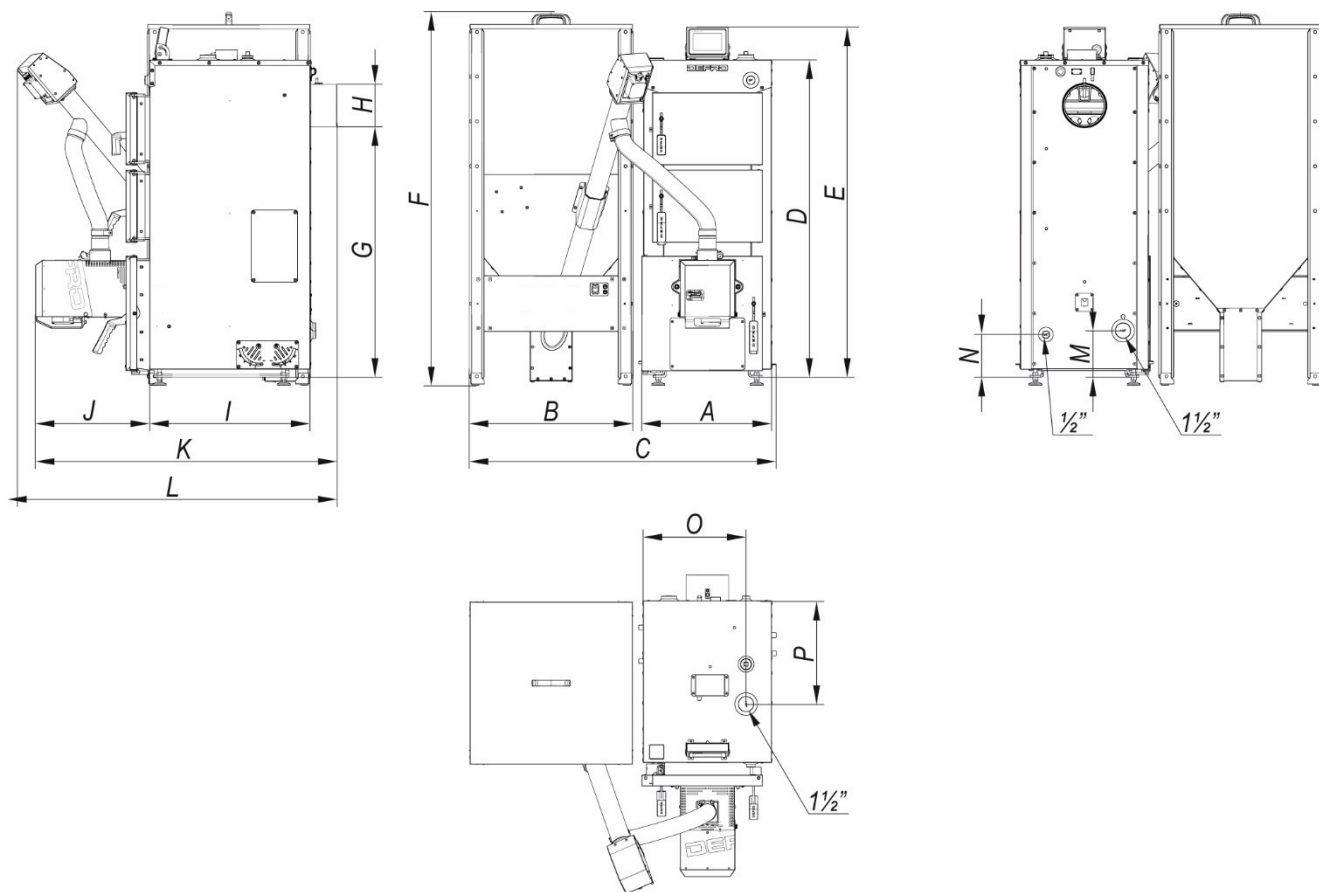
Rysunek 2. Podstawowe wymiary kotła FIREWOOD DUO
