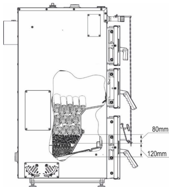
Rysunek 20. Prawidłowe ułożenie paliwa w komorze paleniskowej.
