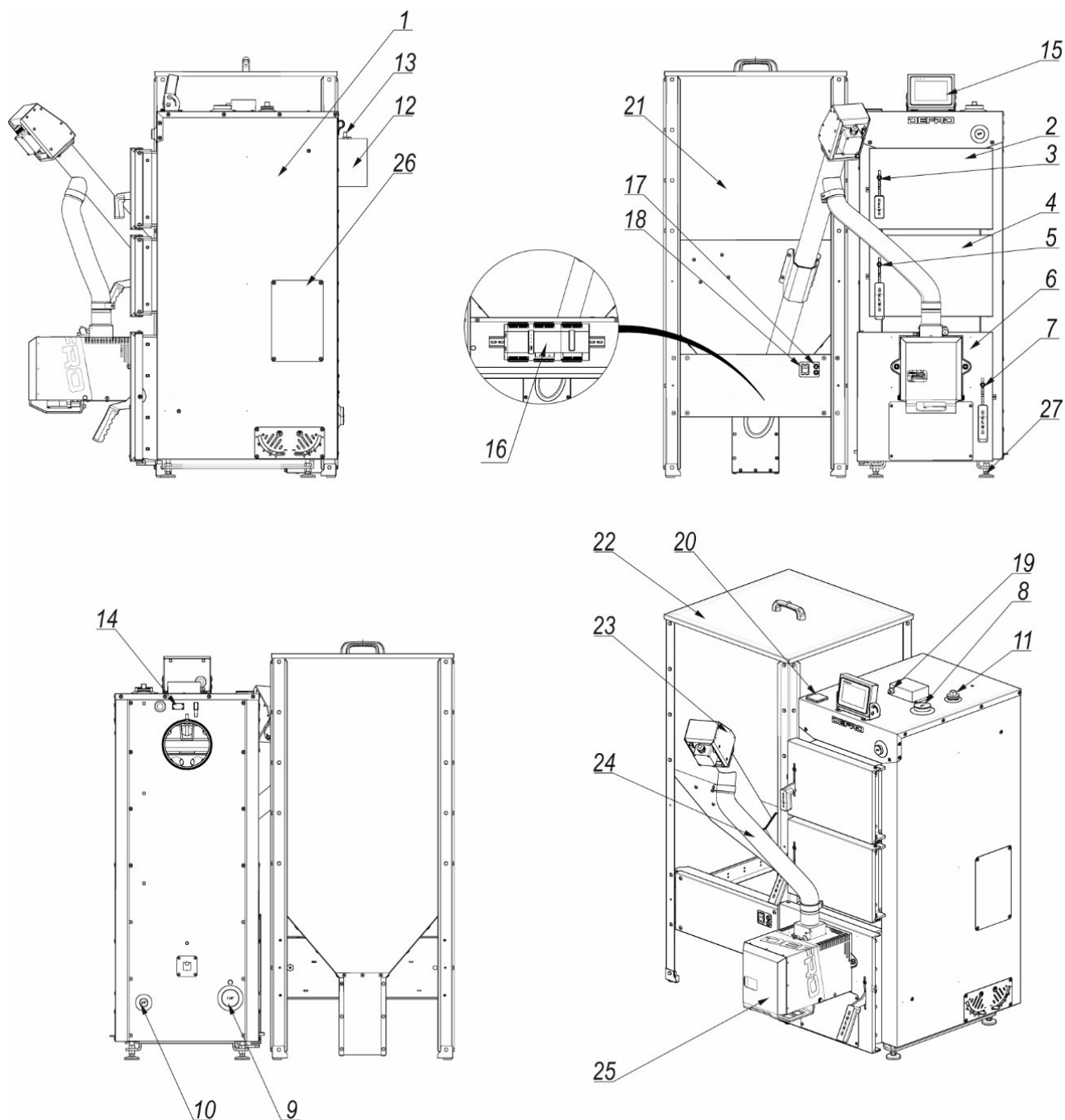
Rysunek 3. Podstawowe elementy kotła FIREWOOD DUO
