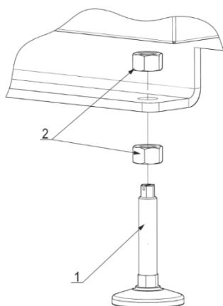
Rysunek 7. Regulowane stopki kotła.
