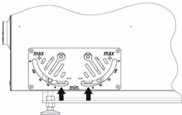
Rysunek 17. Ustawienie przepustnic powietrza wtórnego przed rozpalaniem w kotle.
