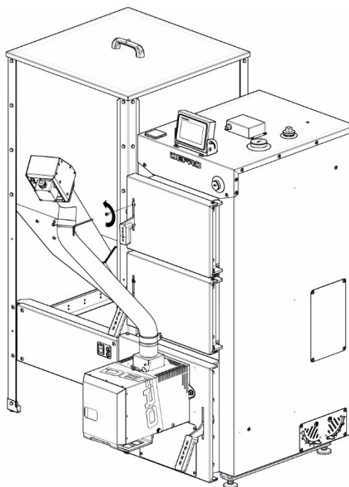
KROK 1. Odkręcić śrubę zabezpieczającą drzwi wyczystne
