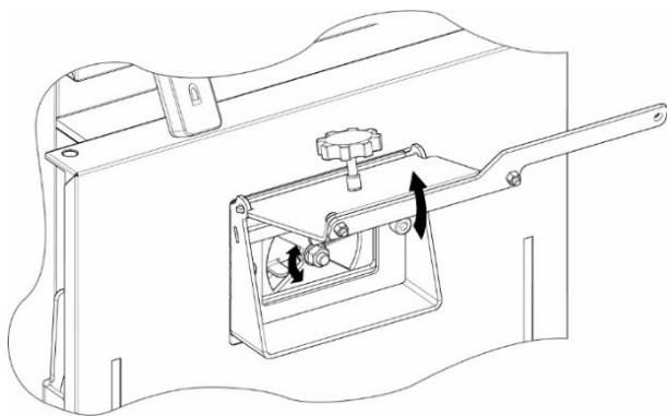
Rysunek 21. Przepustnica regulacji przepływu powietrza.
