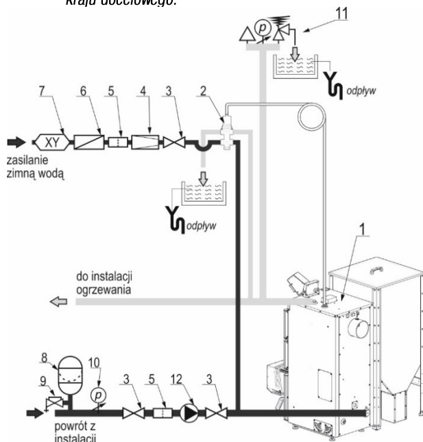
Rysunek 10. Przykładowy schemat zabezpieczeń w układzie zamkniętym FIREWOOD DUO z automatycznym podajnikiem
