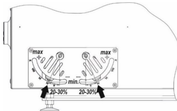
Rysunek 19. Ustawienie przepustnic powietrza wtórnego podczas rozpalania w kotle.
