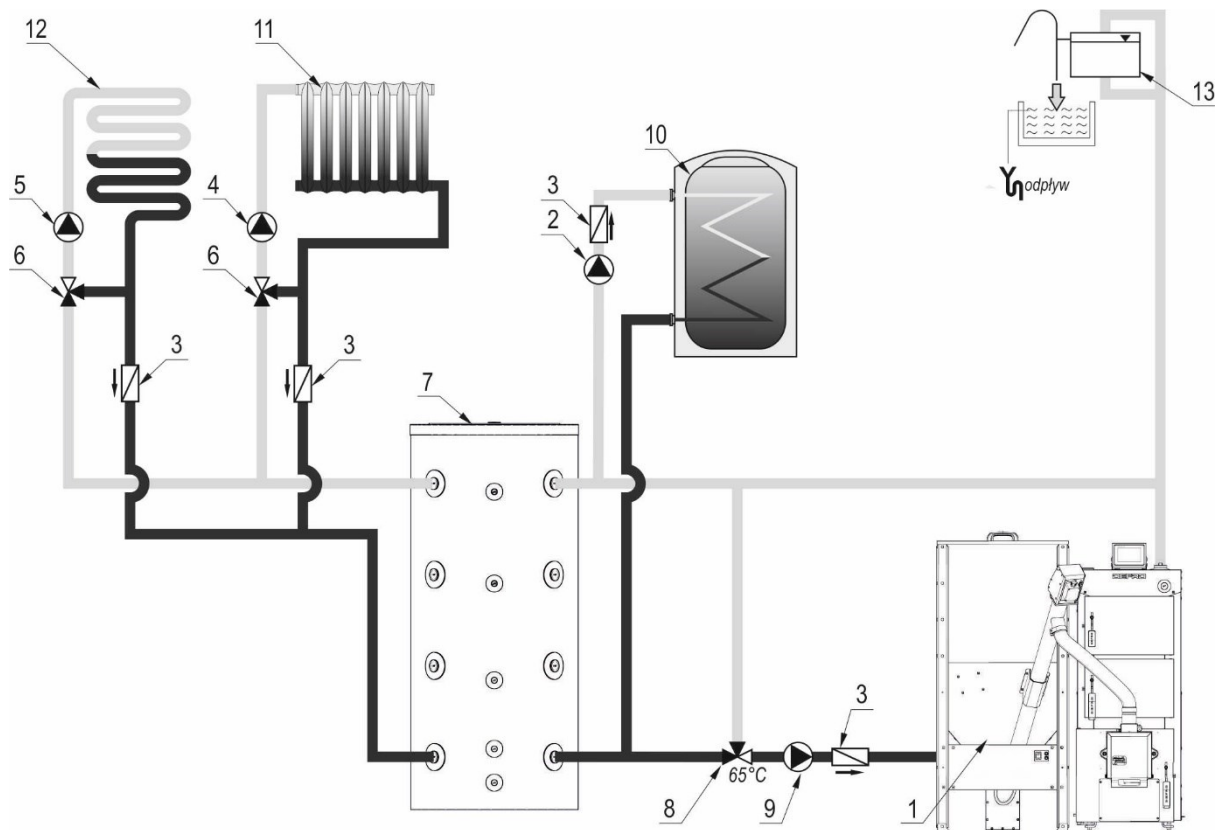
Rysunek 11. Uproszczony schemat instalacji grzewczej systemu otwartego FIREWOOD DUO
