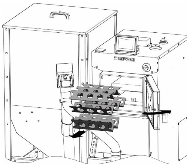
KROK 2. Otworzyć drzwi, wyjąć dolny i środkowy zawirowywacz. Ostrożnie odchylić górny zawirowywacz, wysunąć. Oczyszczyć zawirowywacze oraz powierzchnię wymiany ciepła. Zamontować w odwrotnej kolejności.
