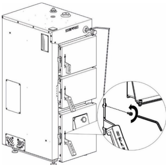
Rysunek 6. Sposób otwarcia drzwi kotła
