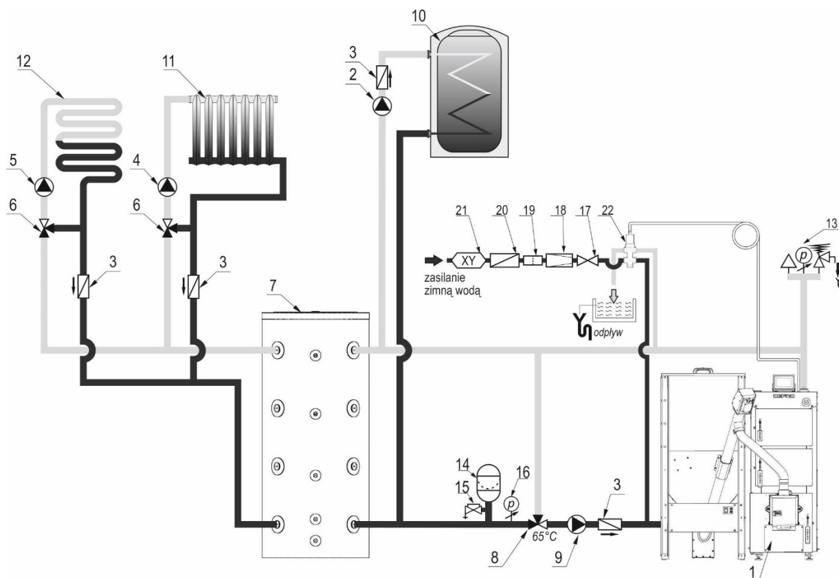
Rysunek 12. Uproszczony schemat instalacji grzewczej systemu zamkniętego FIREWOOD DUO
