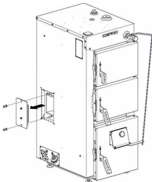
Rysunek 23. Dostęp do wyczystki bocznej
