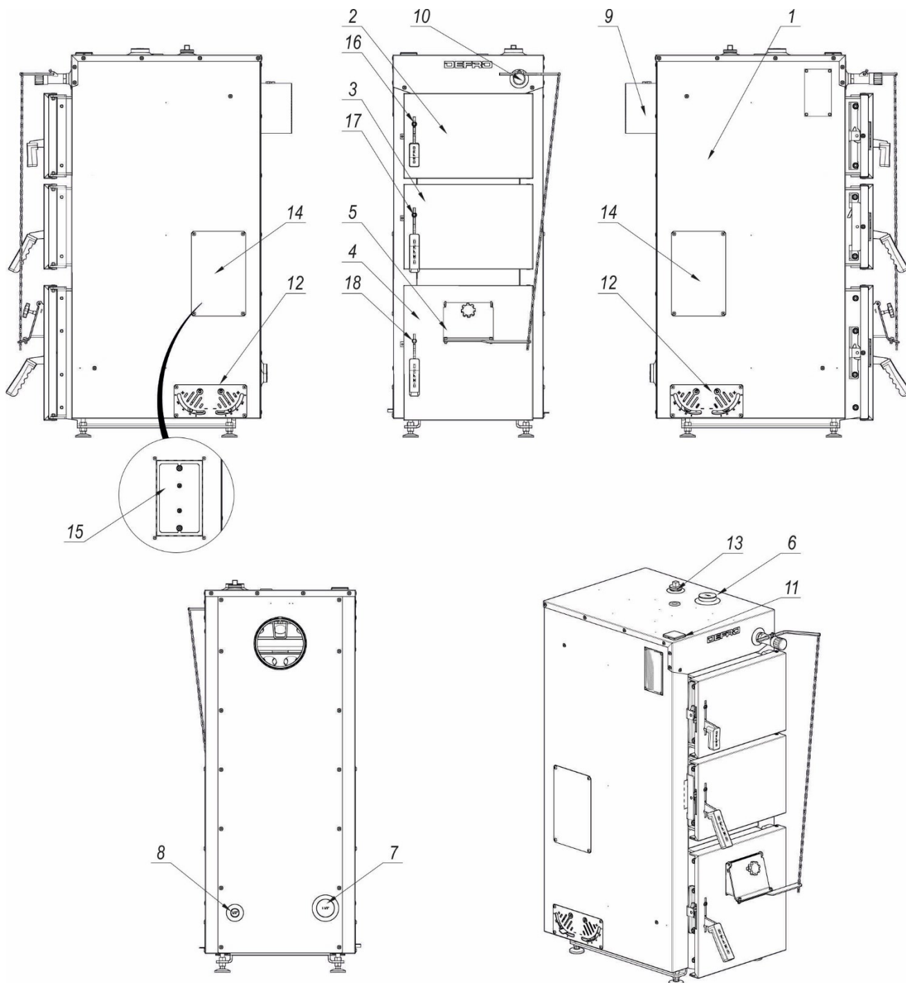
Rysunek 5. Podstawowe elementy kotła FIREWOOD (tryb palenia ręcznego)
