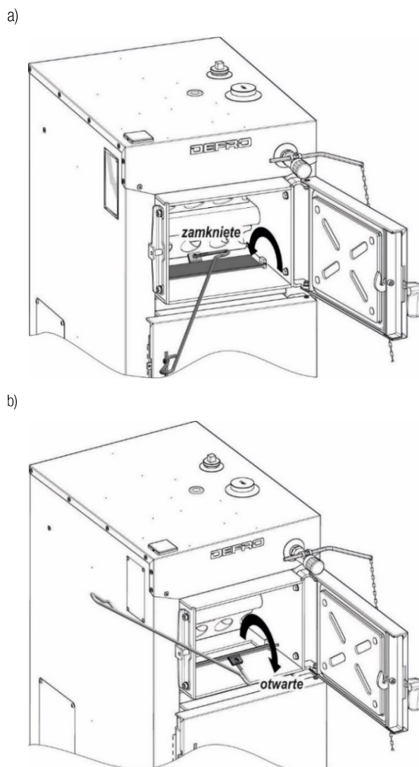
Rysunek 16. Ustawienia klapy krótkiego obiegu.
