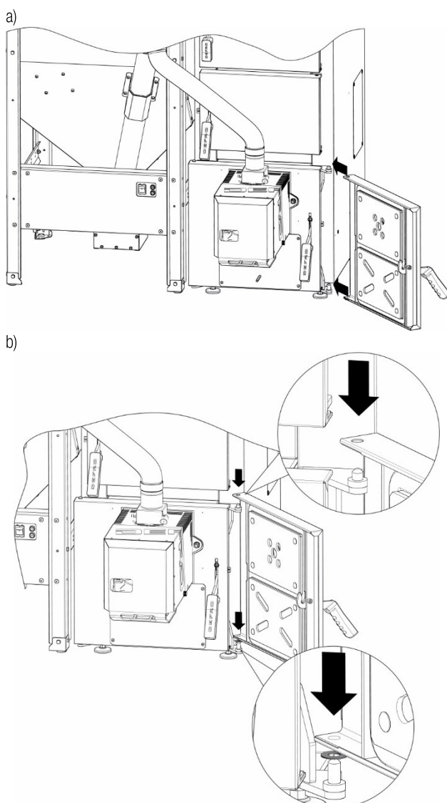
Rysunek 14. Montaż drzwi paleniskowo – popielnikowych
